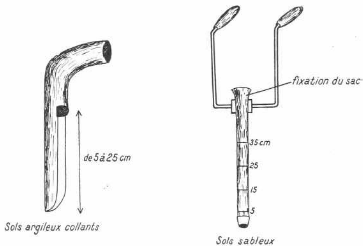
Fig. 9 - Appareillage utilisé pour les prélèvements de sols (échantillonnages agronomiques)
