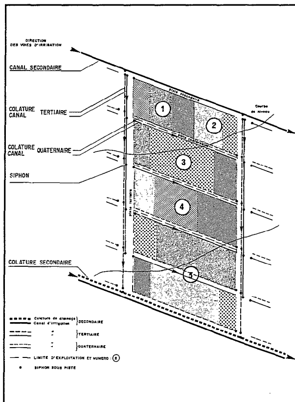
Schéma 2 - BLOC D'IRRIGATION EN TRAME A (accès par l'amont)
