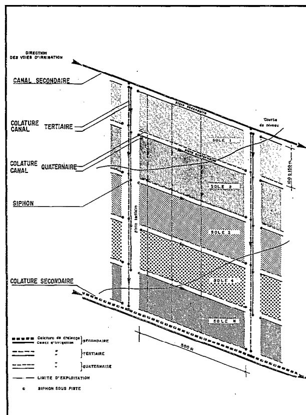
Schéma 1 - BLOC D'IRRIGATION EN TRAME B (accès par l'amont)
