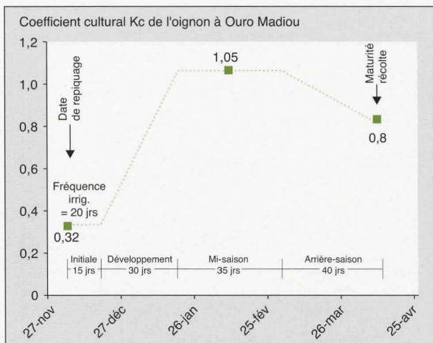
Figure 4. Courbe du coefficient cultural de l'oignon (climat sec, \text{HR}_{\text{min}} faible, vent léger à modéré et \text{ET}_0 phase initiale \sim 3 \text{ mm/jour} ).
