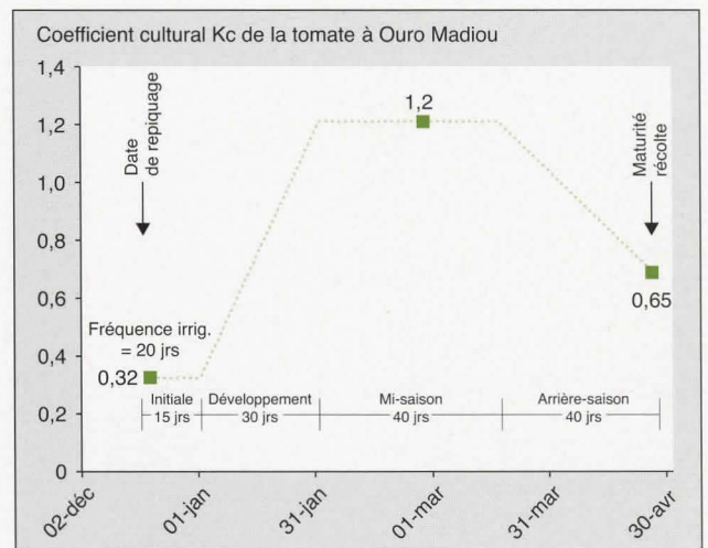
Figure 5. Courbe du coefficient cultural de la tomate (climat sec, \text{HR}_{\text{min}} faible, vent léger à modéré et \text{ET}_0 phase initiale \sim 3 \text{ mm/jour} ).
