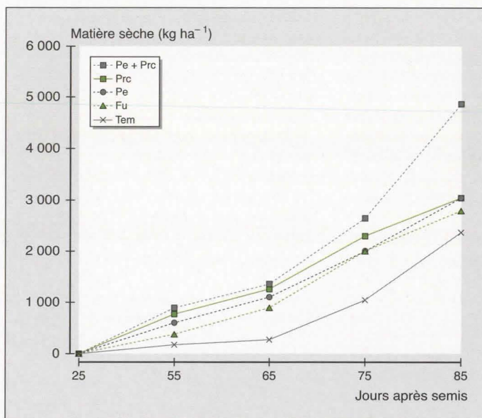
Figure. Effet du fumier sans urine (Fu), du paillage (Pe) et/ou du parcage (Prc) par rapport au témoin (Tem) sur la croissance du mil en 1996.
