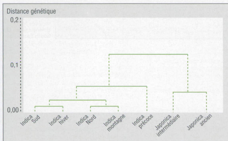
Figure 2. Dendrogramme construit à partir des distances génétiques des groupes de géotypes (variante 1) du riz d'Asie du sud-est.
