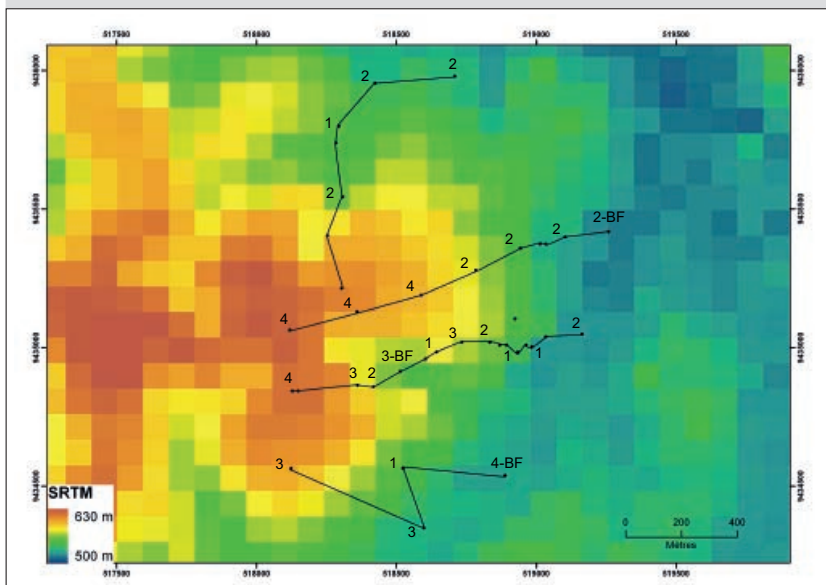
Figure 3. Répartition des types d'horizons sur les transects. 1 = kanga ; 2 = kibuma ; 3 = kiniengi ; 4 = nzielo ; BF = bas-fonds. Les altitudes proviennent d'une image satellite radar SRTM à 90 m de résolution.
