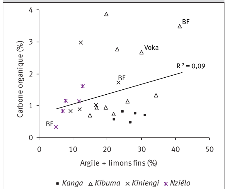
Figure 5. Relation entre le carbone organique et les éléments fins minéraux (argile + limons fins) d'échantillons de surface [0-20 cm].
