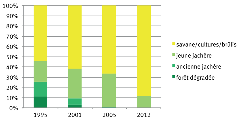
Figure 2. Graphique présentant l'évolution des états de surface dans le finage du village de Kinduala entre 1995 et 2012 (BOULOGNE, 2012).
