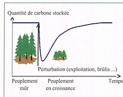
Figure 7. Un exemple de variation de stock de carbone.
