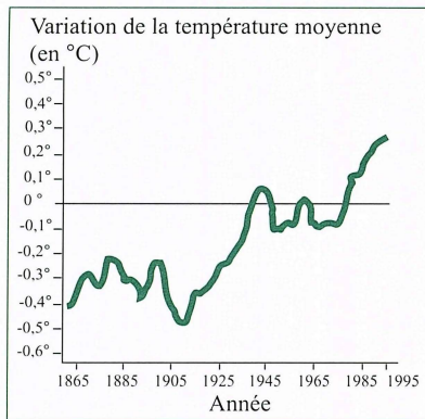
Figure 1. Variation de la température de la terre (d'après SADOURNY, 1992). Variation of the earth's temperature.
