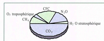
Figure 2. La contribution des principaux gaz à effet de serre au réchauffement de la planète entre 1980 et 1990 (d'après WMO, 1990).
