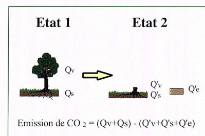
Figure 6. Application de la loi de conservation des éléments pour estimer un flux de carbone entre deux états.
