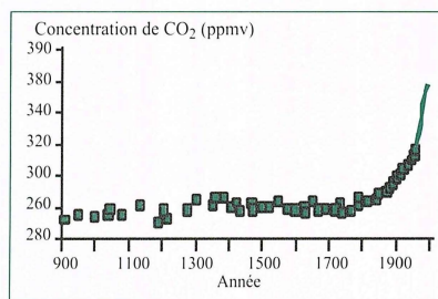
Figure 3. Variation de la concentration de \text{CO}_2 au cours du dernier millénaire (d'après WMO, 1990). Variation in the concentration of \text{CO}_2 over the past millennium.
