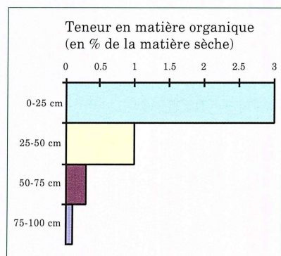
Figure 8. Teneur en matière organique sur un profil de sol (d'après BURINGH, 1984).
