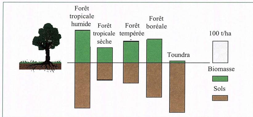
Figure 5. Ordres de grandeurs du stockage de carbone dans la biomasse (aérienne et souterraine) et dans les sols de plusieurs écosystèmes.
