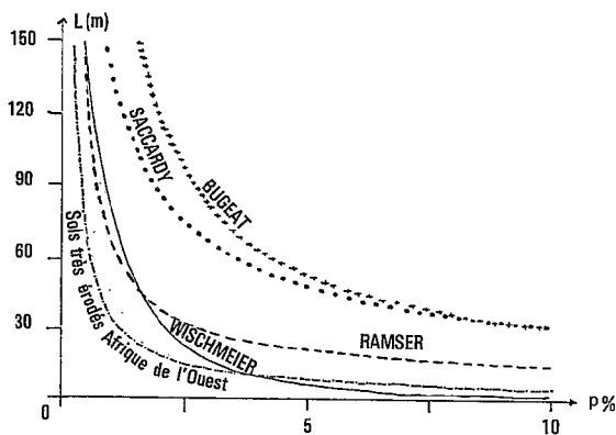
FIG. 5. — Ecartement des dispositifs anti-érosifs.
