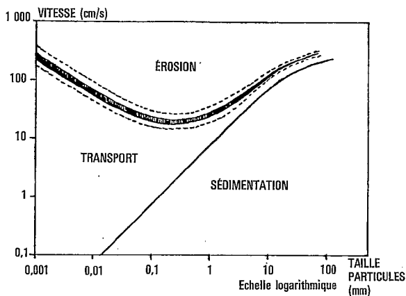
FIG. 3. — Courbes d'érosion et de sédimentation. (Matériau uniforme.) D'après HJULSTRÖM.
