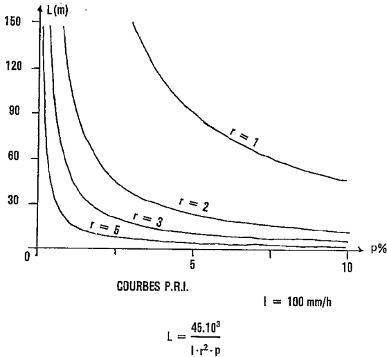
FIG. 4. — Ecartement des dispositifs anti-érosifs.
