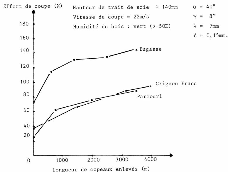
FIG. 6. — Influence de l'usure sur l'effort de coupe pour trois essences guyanaises.
