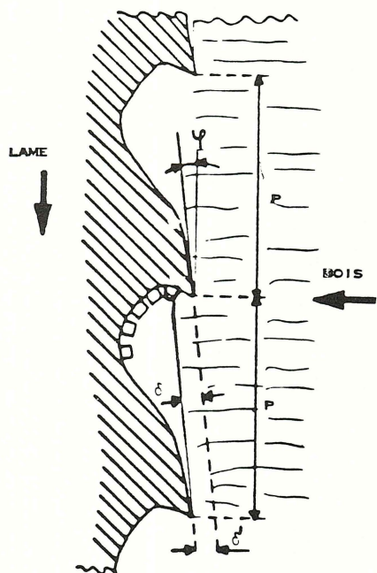
FIG. 3. — Définition des paramètres géométriques caractérisant la denture.
