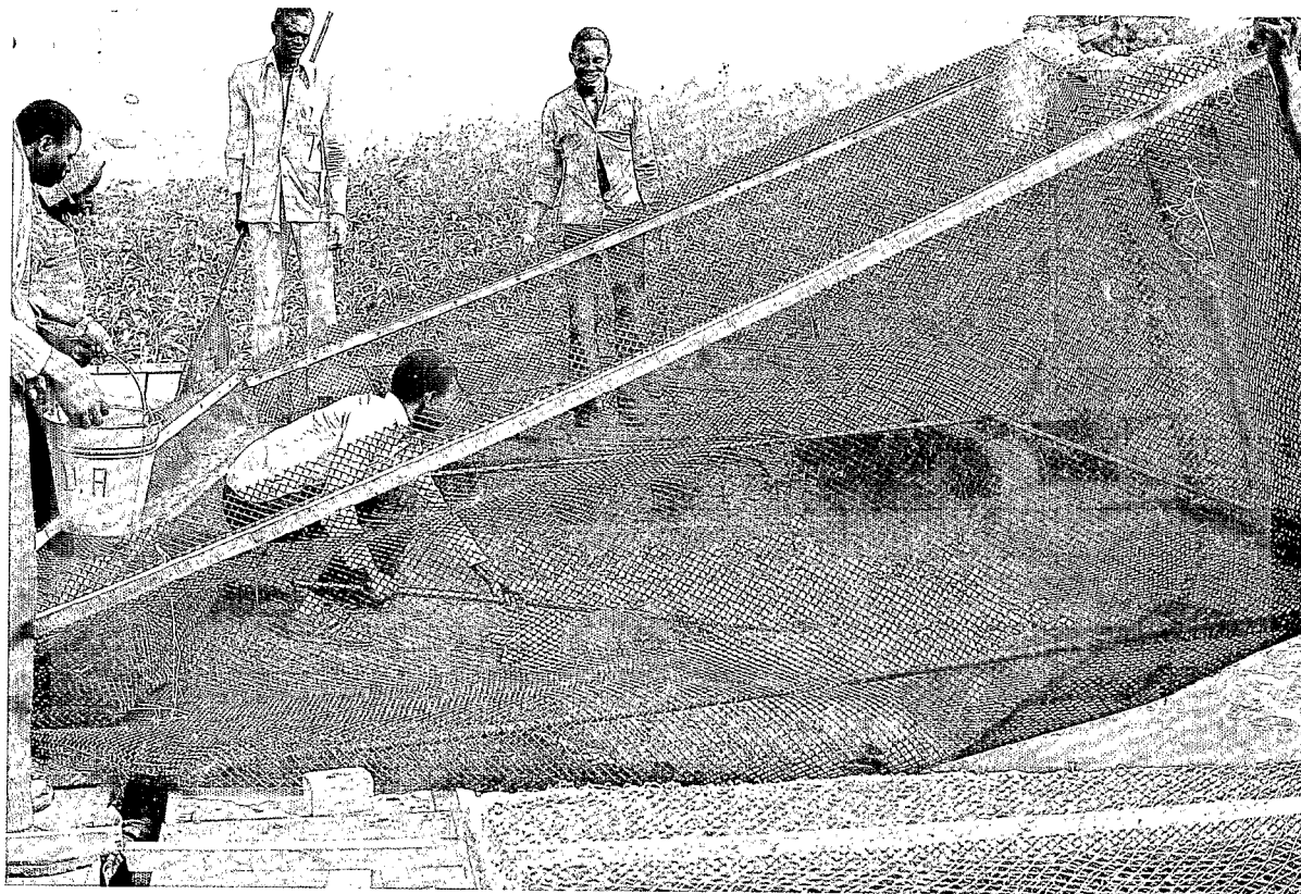
Pêche intermédiaire d'une cage flottante de production de poisson marchand ; au second plan (amont) la plate-forme flottante et la barrière de végétation protégeant contre la force du courant.
