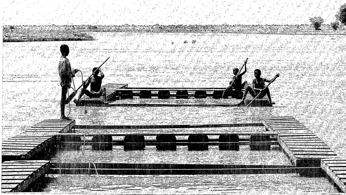
Mise en place des pontons flottants sur le Fleuve Niger (chaque ponton supporte 2 cages de 20 m 3 ou 8 cages de 5 m 3 ).
