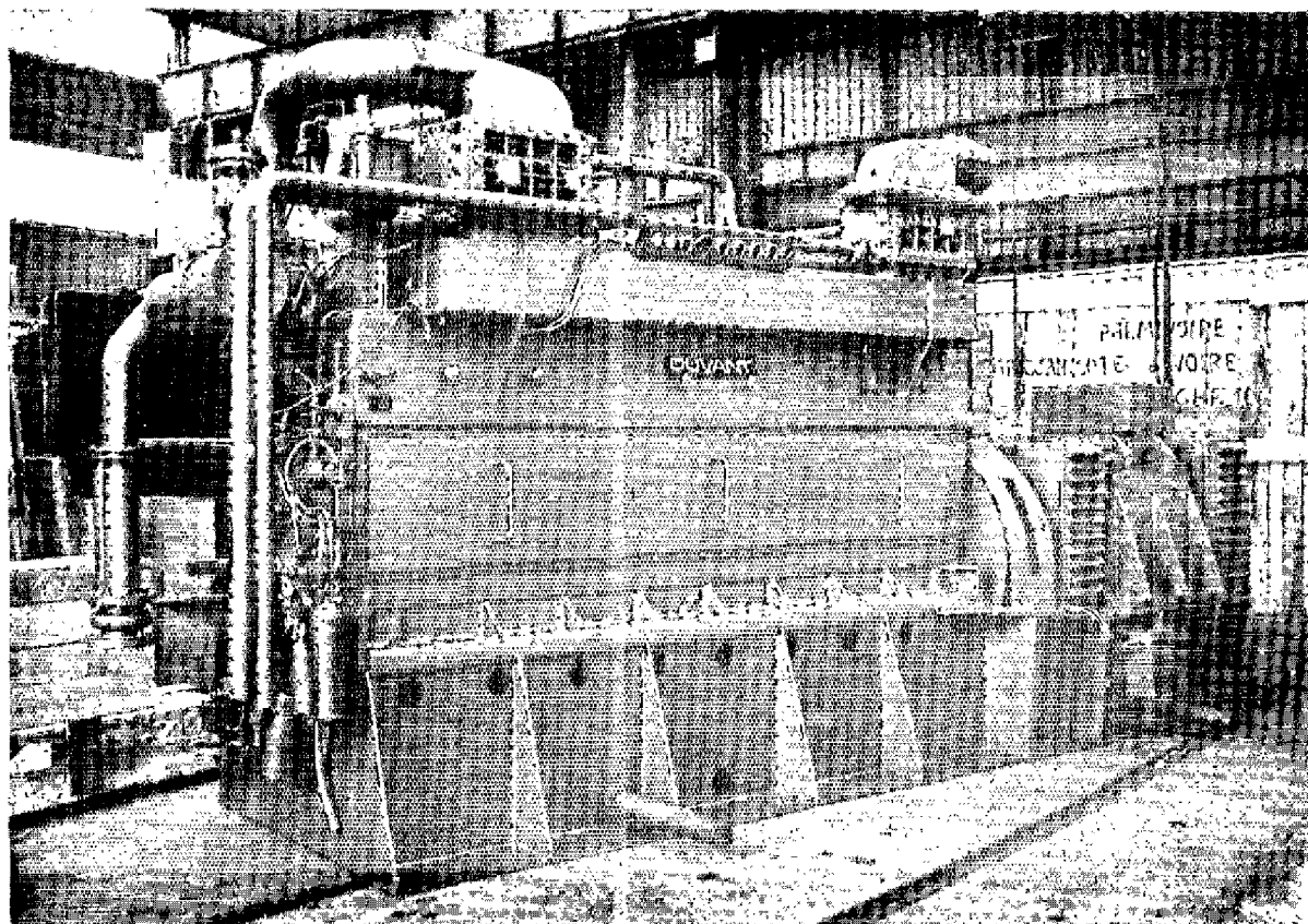
Groupe électrogène DUVANT de 800 KVA - 750 tours.
