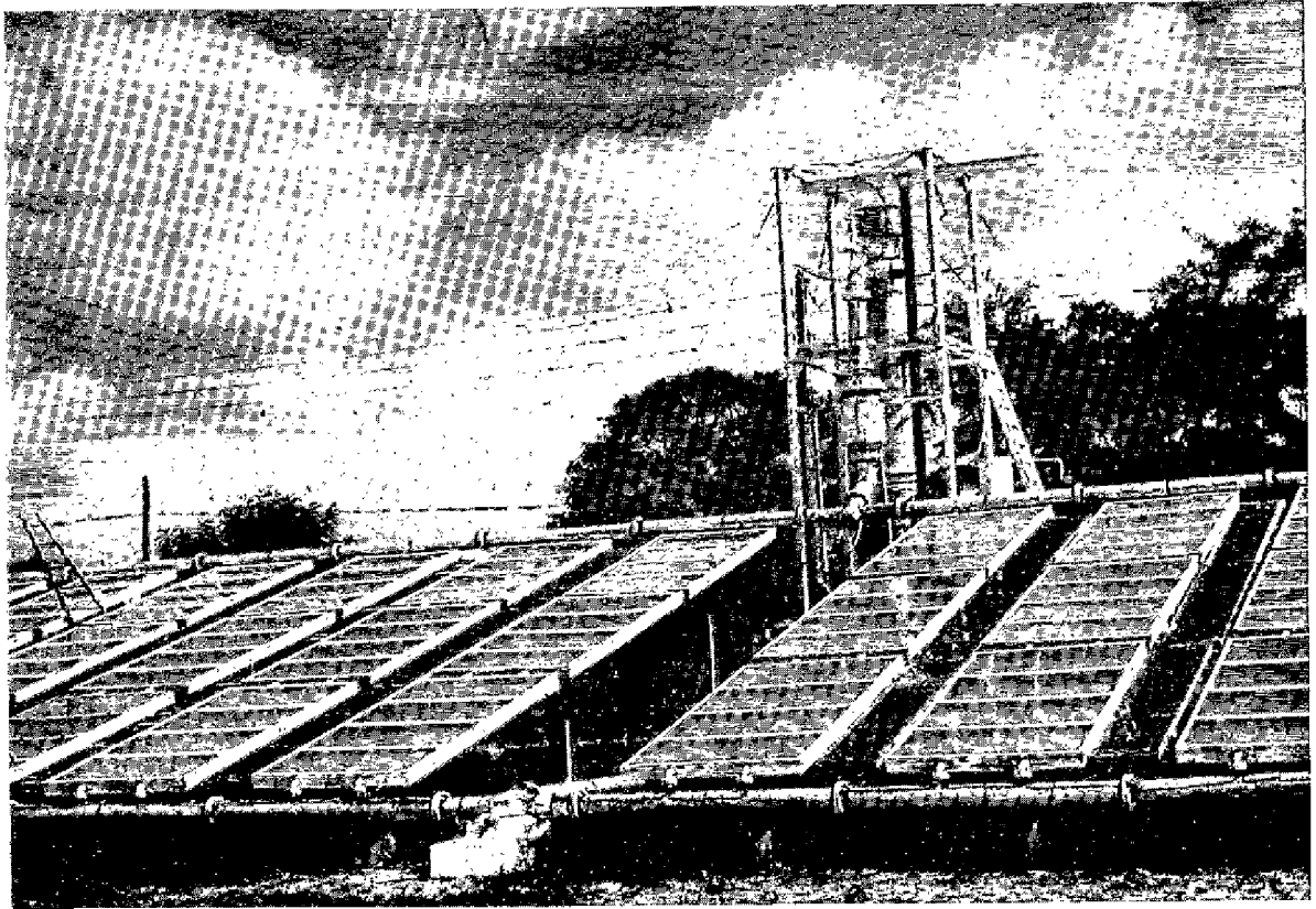
Capter l'énergie solaire, un impératif pour l'avenir du Sahel — Pompe solaire expérimentale à Dakar (Sénégal) — 1976.
