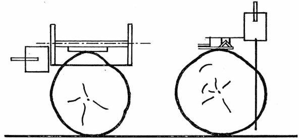
Scie de long à chaîne, type Grandberg.
