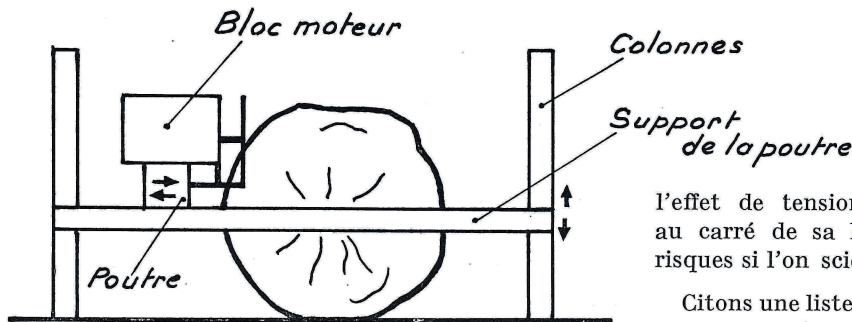
Schéma d'une scie circulaire pour le sciage dans la masse.
