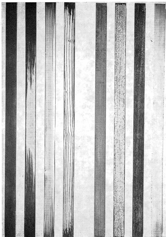
FIG. 3. — Sections longitudinales montrant des pénétrations typiques obtenues avec quatre essences feuillues (gauche) et quatre résineux (droite) :
