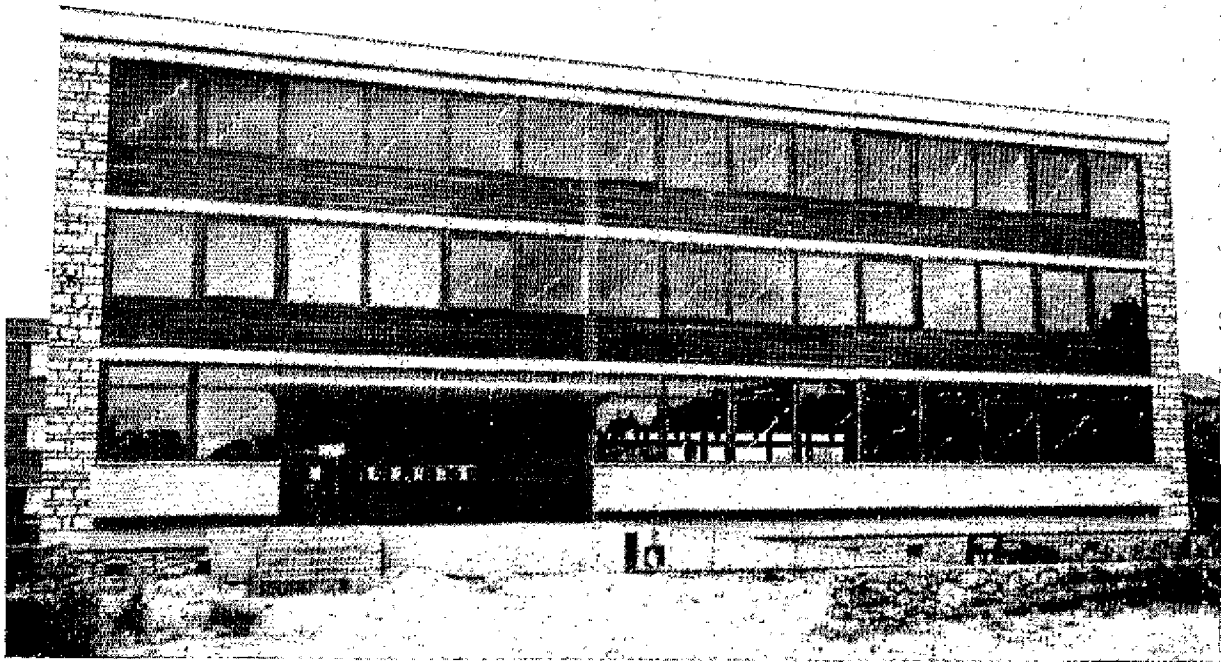
Laboratoires Lerès-Bagneux. Ossature en résineux, fenêtres en Doussié.
