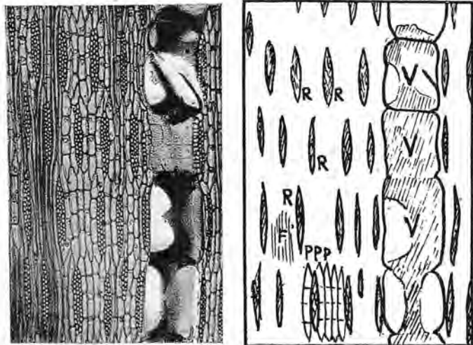
FIG. 2. — Lignes d'étagement ( \times 55 , Afambéou, microphoto C.F.T.F. n° 252). Les éléments sont disposés comme les étages d'une maison : V : élément de vaisseau ; R : rayon ; P : file de 4 cellules de parenchyme ; F : fibres
