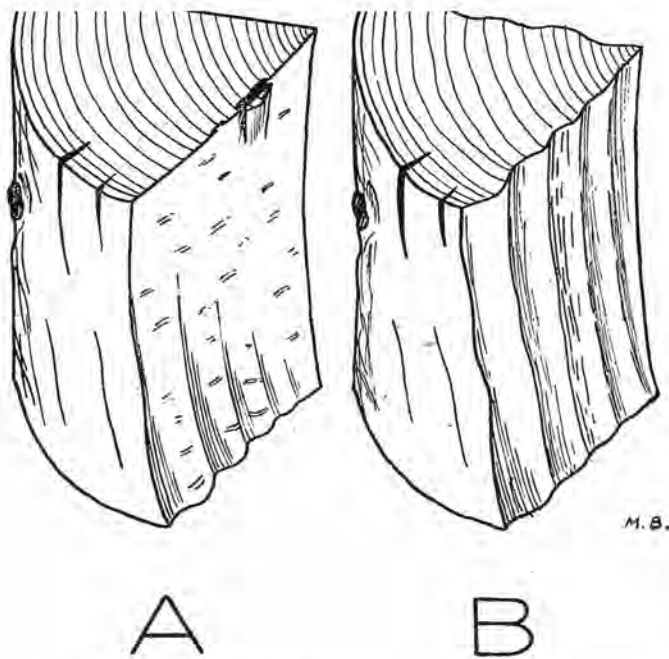
FIG. 5. — Contrefil et torsion du fil. Sur un bois « vrillé » et à contrefil, deux billots ont été obtenus : A par fente et B par éclatement
