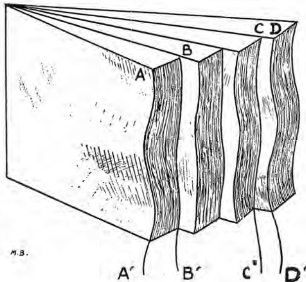
FIG. 9. — Ondulation du fil. Sur ce schéma les éléments ondulent dans des plans tangentiels (AA' et BB' ne sont pas parallèles) et dans des plans radiaux (CC' et DD' ne sont pas parallèles). Si l'ondulation dans le plan radial est peu ou pas marquée, on a un bois ondulé ; si elle est nette, on a un bois madré ou moiré
