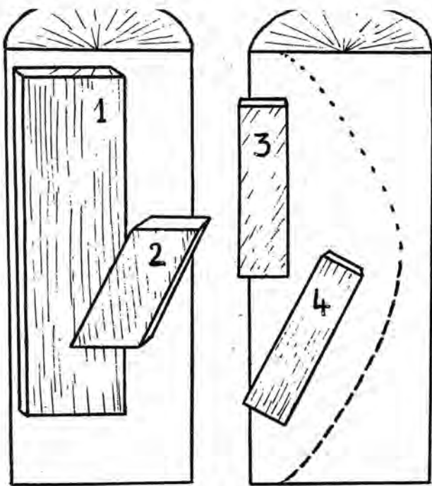
FIG. 14. — Fil et débit. A gauche, de droit fil ; à droite, fibre torse ; une fibre a été schématisée par des tirets en avant du plan de section du rondin et par des pointillés en arrière de ce plan. 1 est de droit fil, 2 est un débit oblique, 3 est un débit d'un bois de droit fil à fil contre-taillé sur un bois à fil tors, 4 est un débit oblique sur un bois à fil tors : on ne peut dire que 4 est de droit fil car ses fibres ne sont pas parallèles à l'axe de l'arbre
