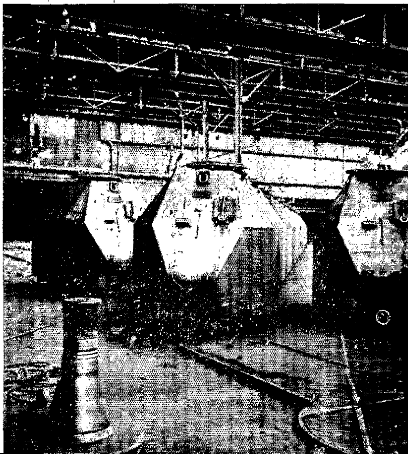
Train de waggonnets étouffoirs à la S.P.C.C.
