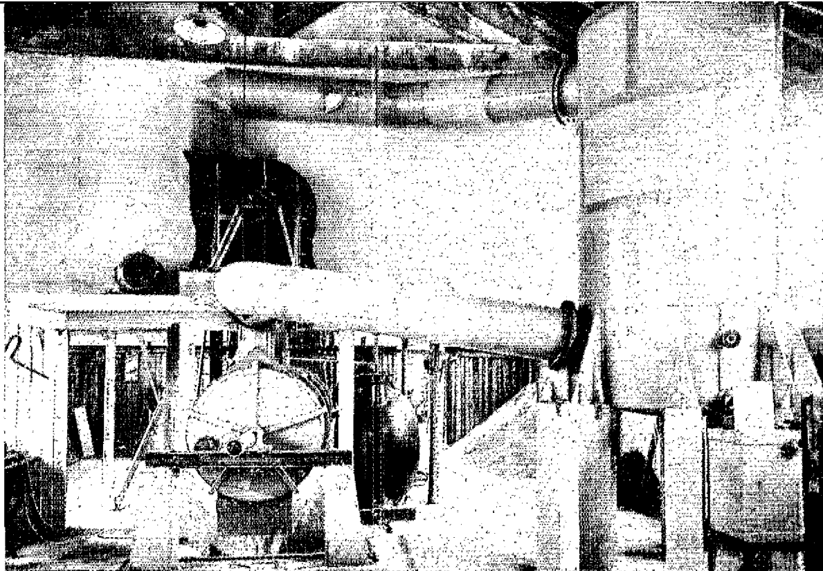
Vue de la tour d'hydrolyse du bois de l'usine de la Société « Hydrolyse et Dérivés » d'Alençon travaillant par le procédé Hereng
