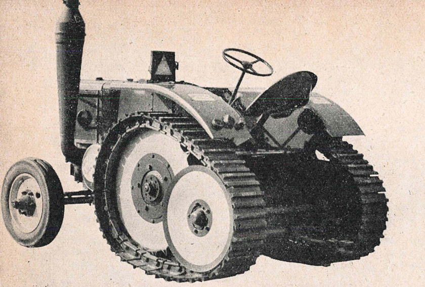
Tracteur Vierzon équipé de la semi-chenille « Roadless » l'un type qui, depuis plusieurs années, donne satisfaction en Angleterre
