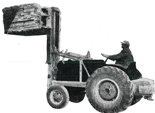
Tracteur à roues équipé en Lift-Truck
